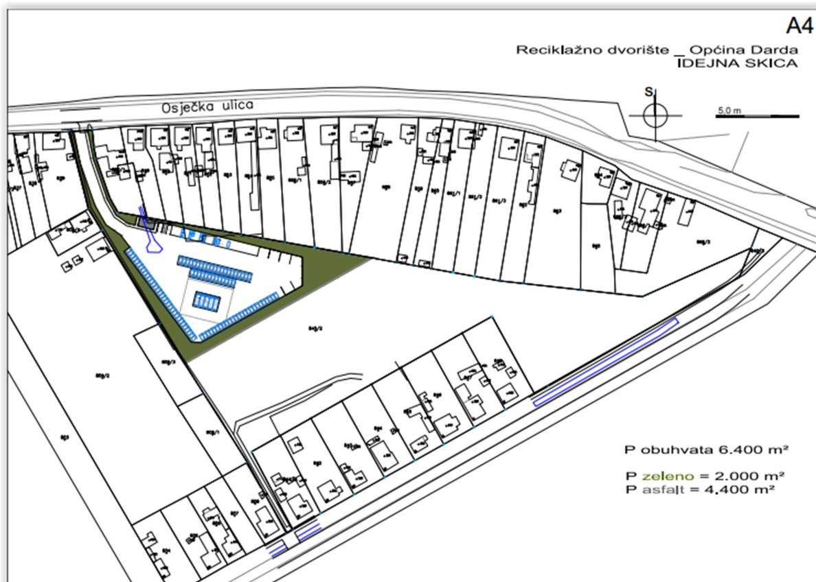
Slika5: Idejno rješenje – reciklažno dvorište Općina Darda (Hidroplan d.o.o. Zagreb)
